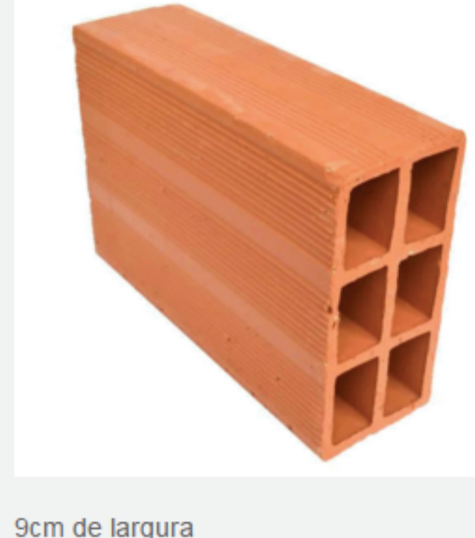
Bloco 9x19x24
